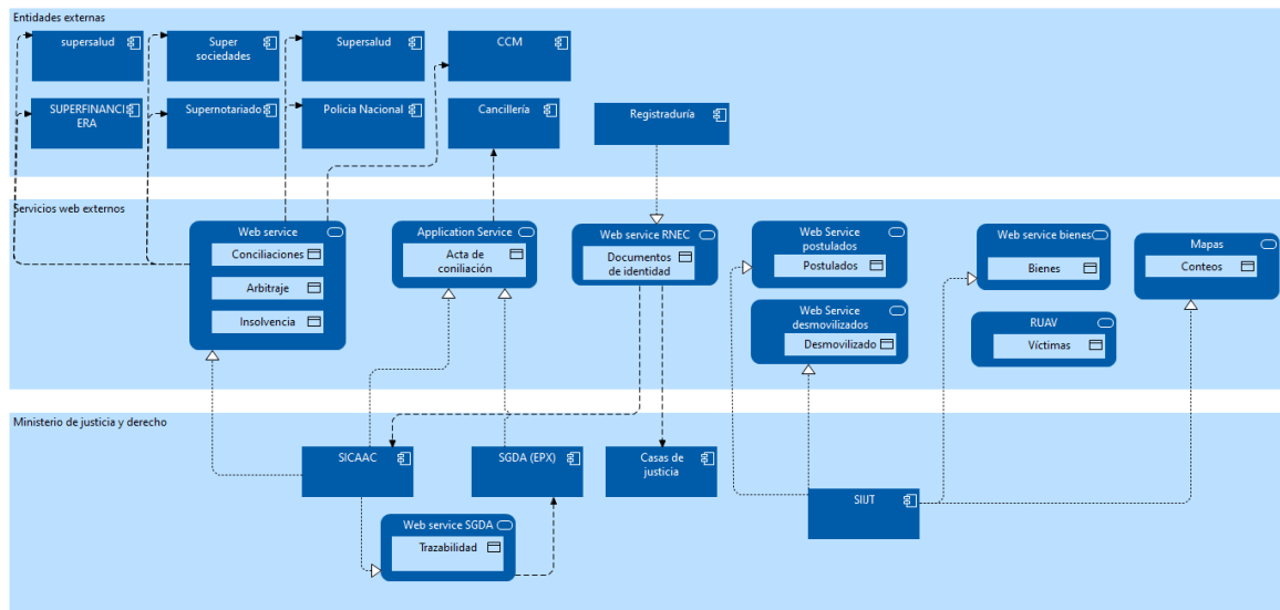
Ilustración 53 Esquema general de interoperabilidad
